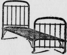
Nr. 7511. Aus 33 mm Stahlrohr, mit Prima Kettennetzmatratze u. Messingverzierung, auf Rollen, weiss lackiert Größe 195x95 cm
