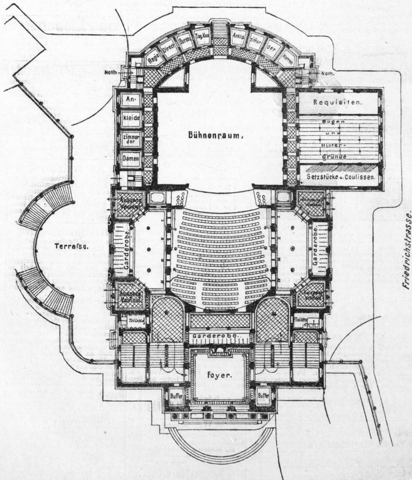
Hauptgrundriß.
