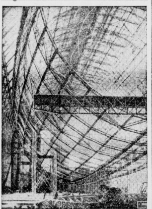
Das Gerippe des Helium-Geppelins.
