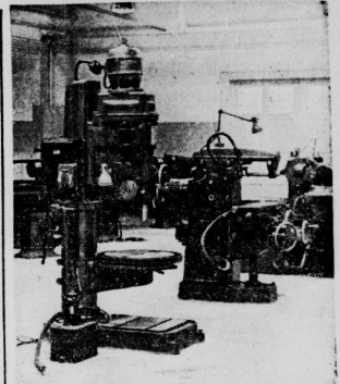
Dreherei und Werkzeugmaschinen. (Bild: Stadtbauamt.)
