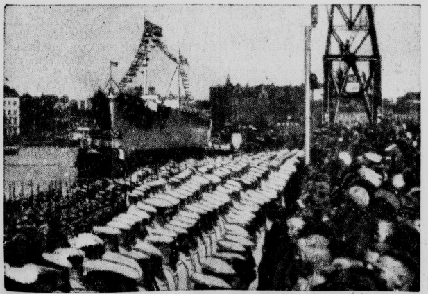
Der feierliche Stapellauf auf der Kieler Germaniawerft Im Beisein des Reichsverwesers v. Horthy und des Führers läuft der neue deutsche Kreuzer „L“ den Frau v. Horthy auf den Namen „Prinz Eugen“ getauft hatte, unter dem Jubel der Menge glatt vom Stapel. (Scherl-Bilderdienst-M.)
