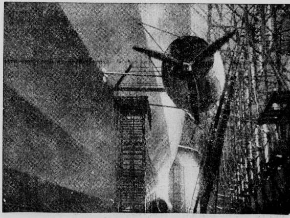
Neueste Aufnahme des neuen Zeppelins Unser Bild zeigt einen Blick auf eine Motoren gondel des Zeppelins in der Halle. (Scherl-M.)
