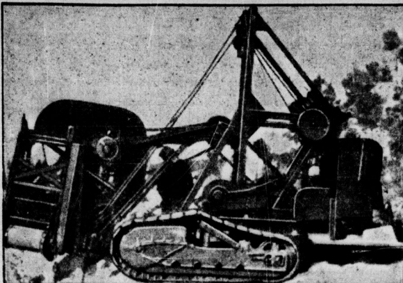
Eine Riesenmaschine, mit der man in den Korallenfelsen Gräben für die Rohrleitung für das Erdgas bohrt
