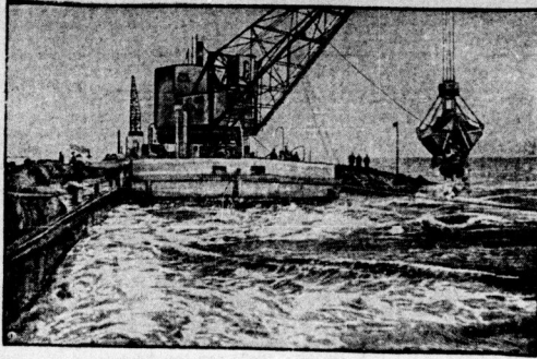
Dieses Projekts sind mit etwa einer Milliarde Mark veranschlagt. — Unter Bild zeigt einen der zahllosen Greifbagger, die in ununterbrochener Arbeit den Damm aufschichten. Die Trockenlegung ist für die Arbeiter außerordentlich gefährlich und schmerzhaft.
