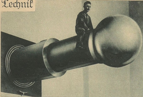
Eine eigenartige elektrische Anlage befindet sich auf dem Hochspannungs-Versuchsfeld der AEG in Berlin-Oberschöneweide, auf der als der größten derartigen Anlage in Europa zurzeit 1 Million Kilowatt konzentriert werden können. Auf dem Bild ist die Einführung der Hochspannungsleitung in das Laboratorium ersichtlich. Um den mit Hochspannung geladenen Pol gegen Koronaverluste zu schützen, hat man ihn als Kugel von 1 Meter Durchmesser ausgebildet. Phot. Scherl
