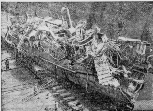
Das „Merkur“-Wrack — ein Bild des Grauens. Wrack im Kaiserdock in Bremerhaven.
