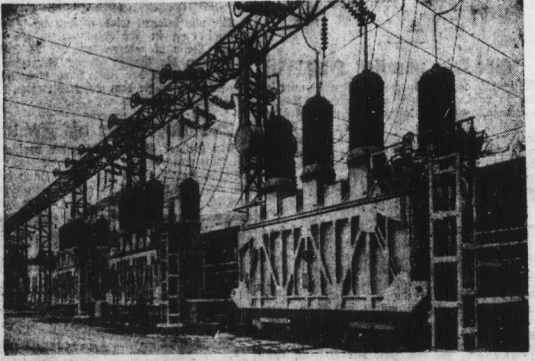
Einige der neuen Transformator des Rheinisch-Westfälischen Elektrizitätswerkes in Braunweiler bei Köln.
