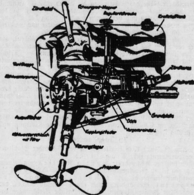
1 1/4-PS-Seitenbordmotor (König) (teilweise geschnitten)
