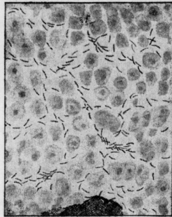
Tuberkelbazillen, die gefährlichsten Bürger der Menschheit (1000fach vergrößert).
