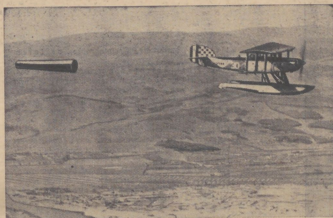
Englisches Wasserflugzeug mit einer beweglichen Zielscheibe, deren Haltetau von dem Flugzeug gerade abgerollt wird. Dieses bewegliche Ziel, das aus dem Schwanz des Flugzeuges herausgelassen wird, wird in einem Abstand von etwa 1,6 km hinterhergeschleppt. Der große Abstand gilt als Vorsichtsmaßregel, damit das Schleppflugzeug von den Schießflugzeugen nicht beschädigt wird.
