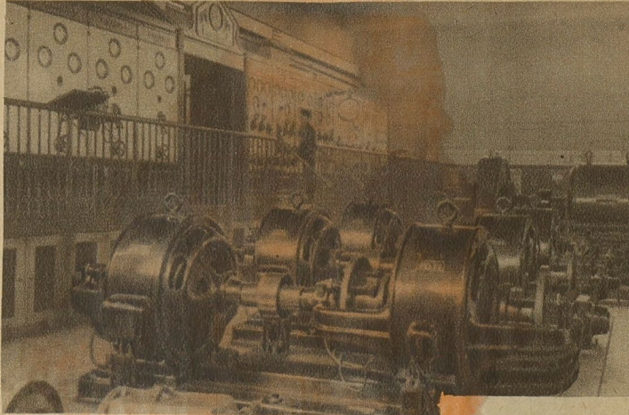
Sämtliche Aufnahmen von Photo Blick auf die Schalttafel der Kraftanlage; im Vordergrund 3 Poulsen-Umformer für 1000 Volt Gleichstrom für Lichtbogen sender
