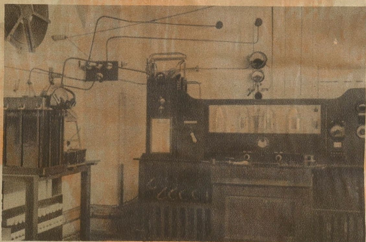
Der Unterhaltungsrundfunk-Sender, der die Vorträge des Volkshauses Berlin auf Welle 475 verstärkt weitersendet (5 KW.)
