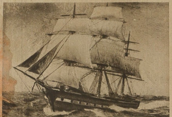
Der Segler „Deutschland“ Phot. R. Sennedé das erste Schiff der „Hapag“ aus dem Jahre 1848
