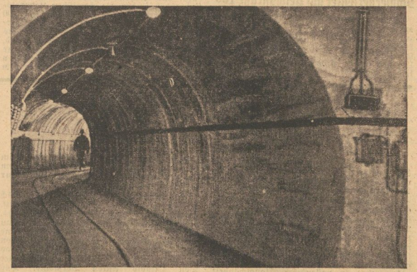
Der neue dokumentarische Film „Der Westwall“ schildert eindrucksvoll die technischen Einzelheiten dieser Mauer aus Stahl und Beton. Hier sehen wir einen Gang mit Beförderungsgleisen in einem der Werke
