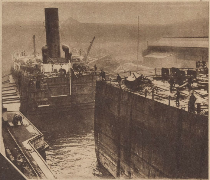
Eine einzigartige „Schiffs-Operation“. Auf einer englischen Werft wird gegenwärtig ein Titan-Dampfer „Cadillac“ repariert. Das Schiff ist dazu in drei Teile geschnitten worden, damit in den mittleren Rumpf Erfschilde eingezogen werden können. Die Aufnahme ist in dem Augenblick gemacht, als das Mittelstück des Dampfers (rechts) abgeschleppt wird Semmede
