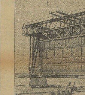
Eine gewaltige Schleusenkammer im Bau.
