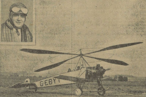
Das eigenartige Windmühlen-Flugzeug. Oben: Sein Erfinder und Erbauer La Cierba.
