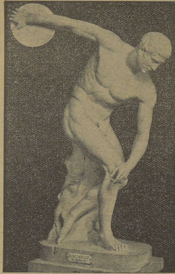
Das olympische Ideal des klassischen Altertums: „Der Diskuswerfer von Myron.“
