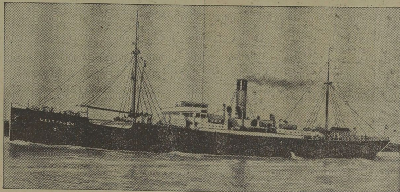
Rechts unten: Frachtdampfer „Westfalen“ des Norddeutschen Lloyd, der von der Luftlinie als Flugzeug-Stützpunkt für die Luftpoststrecke nach Rio de Janeiro umgebaut wird. Der Dampfer erhält ein Heißes Schlepppegel und eine Katapultanlage.
