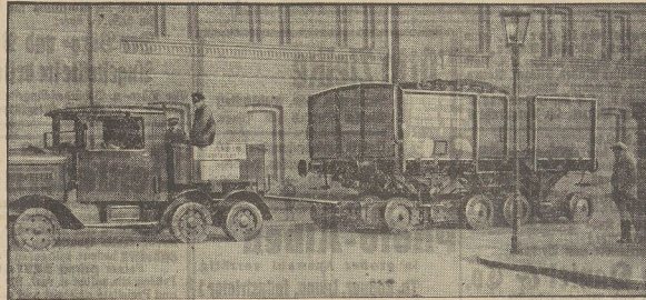
Dieses neue 16rädige Fahrzeug wurde von der Reichsbahn jetzt in Viersen im Rheinland in Dienst gestellt.
