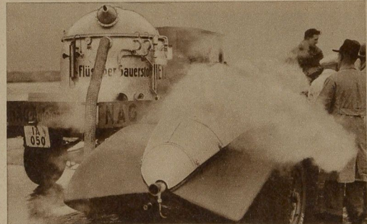
Raketensauto tankt flüssigen Sauerstoff. Auf dem Berliner Flughafen wurde neulich ein neuer Rüststoff-Kraftwagen des Obergerieurs Piesch und des Konstrukteurs Hepland vorgeführt. Während die erste Vorführung mißlang, glückte die zweite vollkommen Semme
