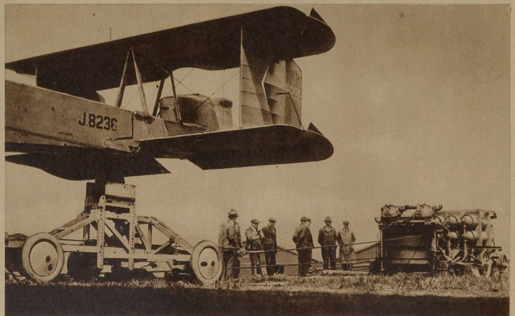
Eine neuartige Katapult-Startvorrichtung für schwere Landflugzeuge wird jetzt in England ausprobiert. Die Betriebskraft wird durch Preßluft von 4000 PS erzeugt. Es können Flugzeuge im Gewicht von über 7000 Kilogramm abgeschleudert werden Sennede
