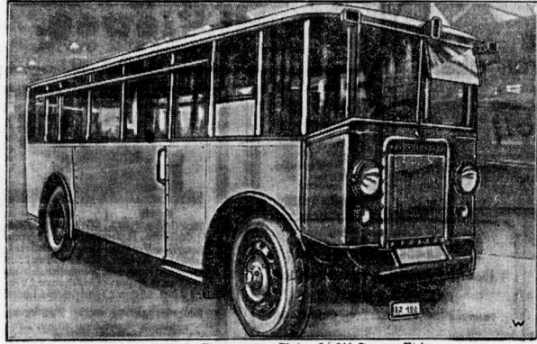
Ein neuerer Mercedes-Benz-Bus mit 34 Tonnen Nutzlasten-Capazität mit Gasantrieb. Der Aufbau weist 38 Sitzplätze und 11 Stehplätze auf. Der Wagen entwickelt eine Geschwindigkeit von 38 bis 46 Kilometern in der Stunde.
