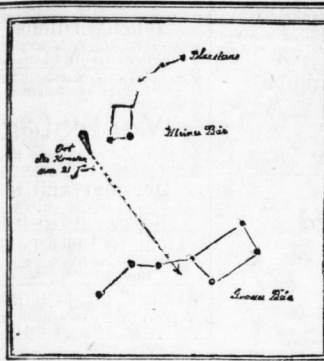
Karte zum Auffinden des Kometen Vostok.
