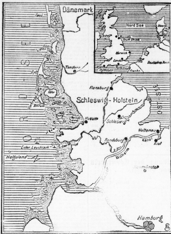
Die Westküste von Schleswig-Holstein. Oben: Die Küsten der Nordsee.
