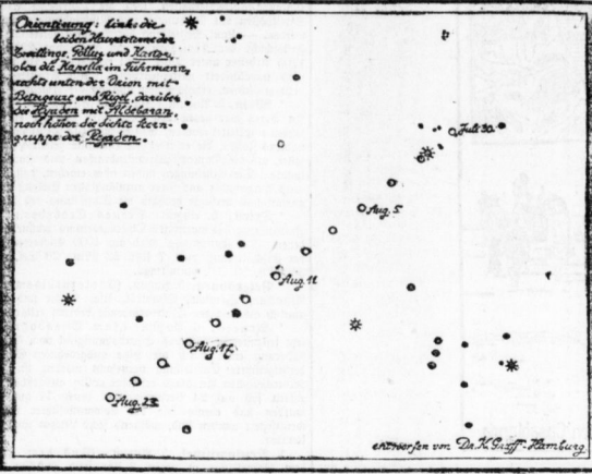
Die Bahn des neuen Kometen.
