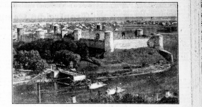
Blick auf die Festung Lwów nach der Einnahme durch die deutschen Truppen Der Festung Narwa gegenüber befindet sich die Festung Lwów, die ebenfalls von unseren Truppen erobert wurde. — Blick über die alten Festungsanlagen der Stadt. Im Vordergrund die von den Bolschewisten gesprengte Brücke. (PK. Schmidt/Scherl-A.)
