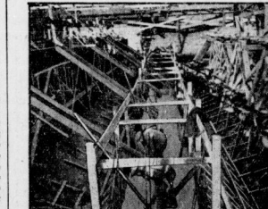
Beim Betonieren der Gosafang-Däme.
