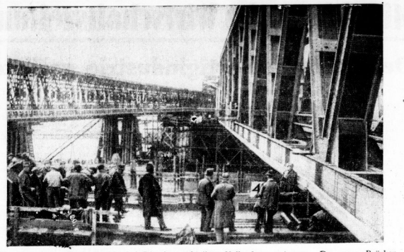
Die neue große Weichselbrücke bei Dirschau geht ihrer Vollendung entgegen. Der neue Brückenkörper wird, wie unser Bild zeigt, in seine endgültige Lage gebracht.
