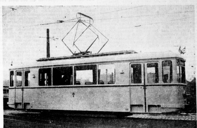
Gesamtansicht des neuen Erriebwagens der hallischen Straßenbahn (Aufnahmen: Giegold Schilling)
