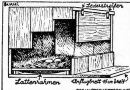
Das Nestkastenmodell zeigt die Konstruktion des Lattenrahmens und der Schwanzflügel, die durch eine Klappe geschützt sind.
