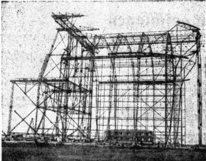
Die Montage der neuen großen Luftschiffhalle
