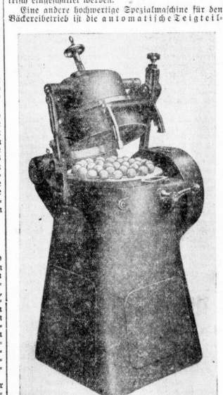
Teigteil- und Wirkmaschine.
