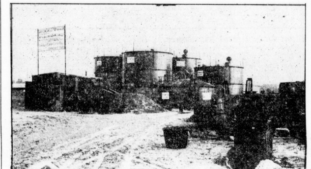
Die fünf 100-cbm-Tanks im Plan.
