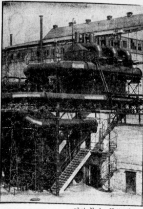
phot. Nachert-Hettstedt. Moderne Technik: Generatoren-Anlage auf dem Mansfeld-Steinwerk.
