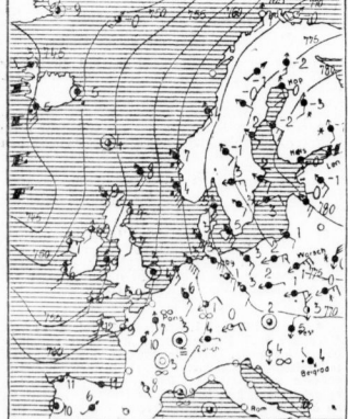
ERKLÄRUNG: Die Wetterkarte zeigt die Wetterlage am 20. November 1931. Die Isobaren sind in Millibaren angegeben. Die Wetterlagen sind durch Symbole dargestellt.
