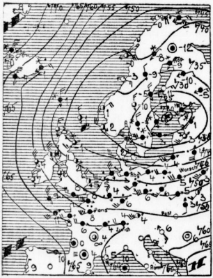
Wetterkarte vom 29. Dezember 1931. Staatliche Wetterdienst der Luftfahrt-Verwaltung.
