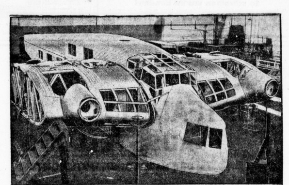
Der Umbau des „D 2000“. Das riesige Dampfkessel-Boilergehäuse, das jetzt eine gewöhnliche Kabinen enthält...
