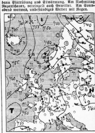
ERKLÄRUNG: Gewitter, Regen, Nebel, Frost, etc. Die Pfeile zeigen die Richtung der Luftbewegung an.
