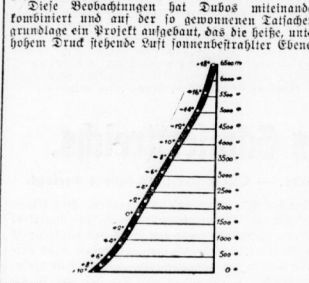
Abb. 11. Wie die Temperatur in der freien Atmosphäre mit zunehmender Höhe abnimmt...
