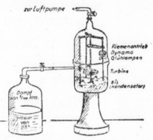
Abb. 18. Die Versuchsanordnung, mit der Claude und Souderet zur Erzeugung von Energie...
