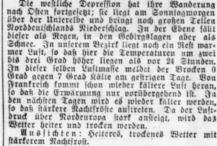
ERLEUTERUNG: Charakteristisches Wetterbild: Hoch über Skandinavien, Tief über Island, Fronten über Nordsee und Ostsee.
