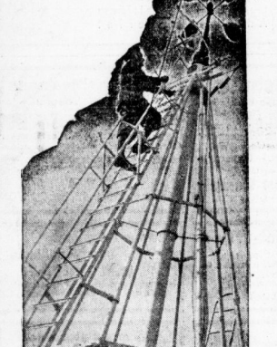
Die Greenbergsche Streu-Antenne für ultrakurze Wellen.
