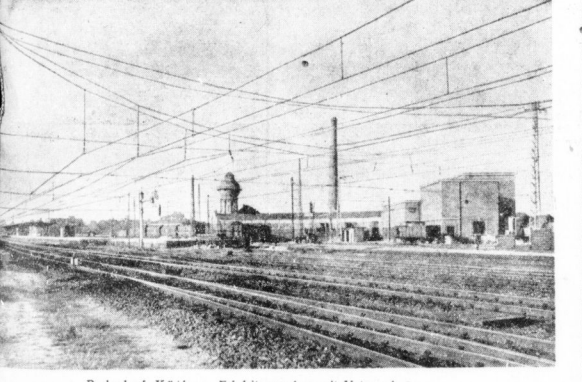
Bahnhof Köthen, Fahrleitungsanlage mit Unterwerk
