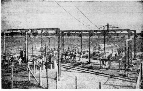
Unterwerk Marke, Freileitungsstelle
