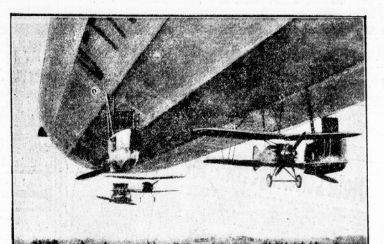
Luftschiff R. 33 mit einem daran hängenden Kampfflugzeug.
