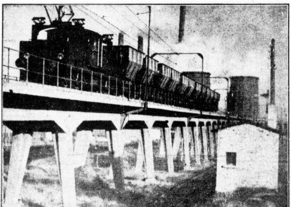
Elektrische Förderbahn, die seit Jahren notwendig wurde, da die Gruben sich ständig weiter in die Land...
