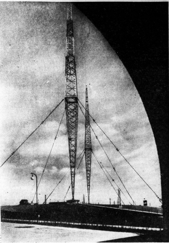
Fischbauchantenne und Relektormast des Wiener Senders
