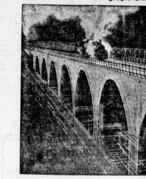
Der neue Nobena-Abfuhr an der Höllebahn im Schwarzauer. Die implannte Brücke hat neun Bögen mit 20 Meter lichter Weite und ist insgesamt 224 Meter lang. ...
